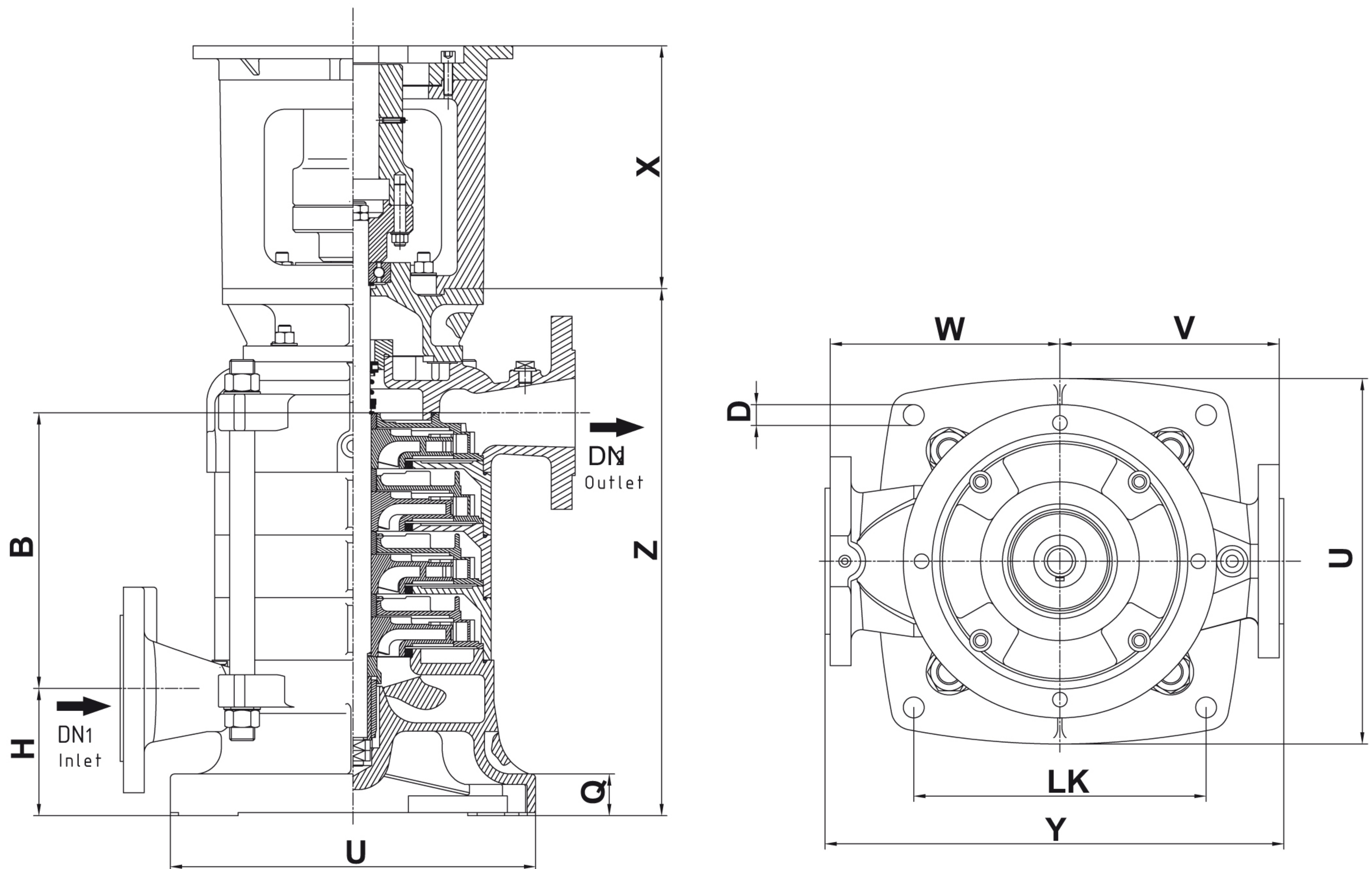
جدول ابعاد پمپ های WKLV4 ,WKLV ( 32-65 )
