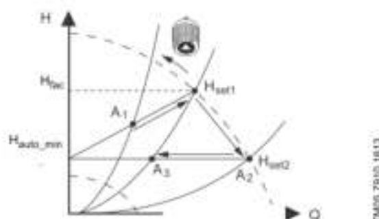
Fig. 50 AUTO ADAPT
