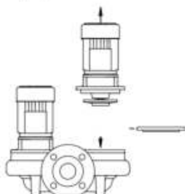
Fig. 174 Blanking flange
