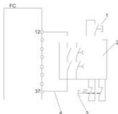
Fig. 162 STO wiring
