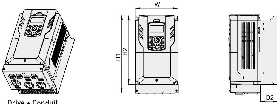
Drive + Conduit
